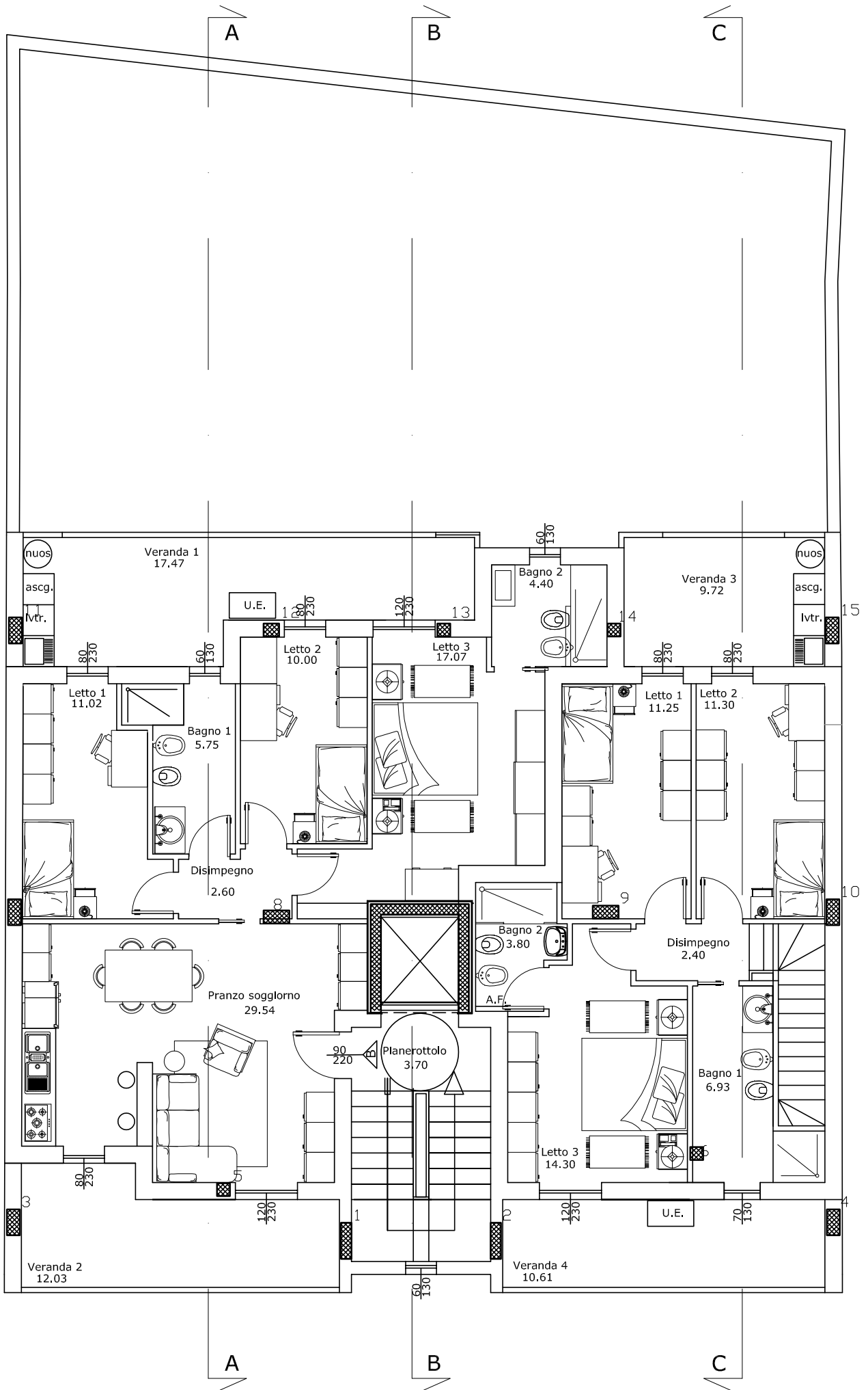
Pianta Piano primo arredata sc. 1:100
