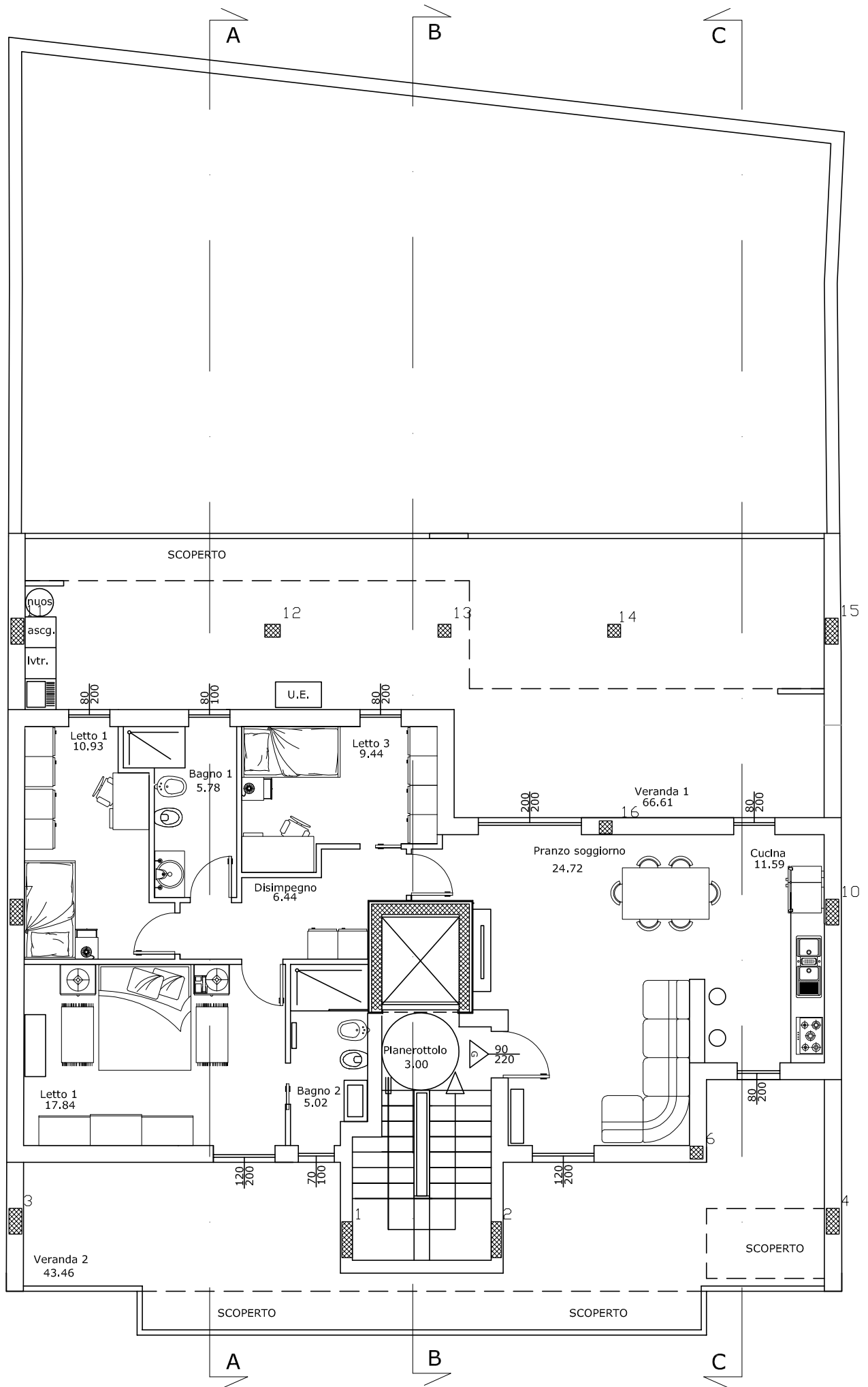
Piano quarto arredata sc. 1:100
