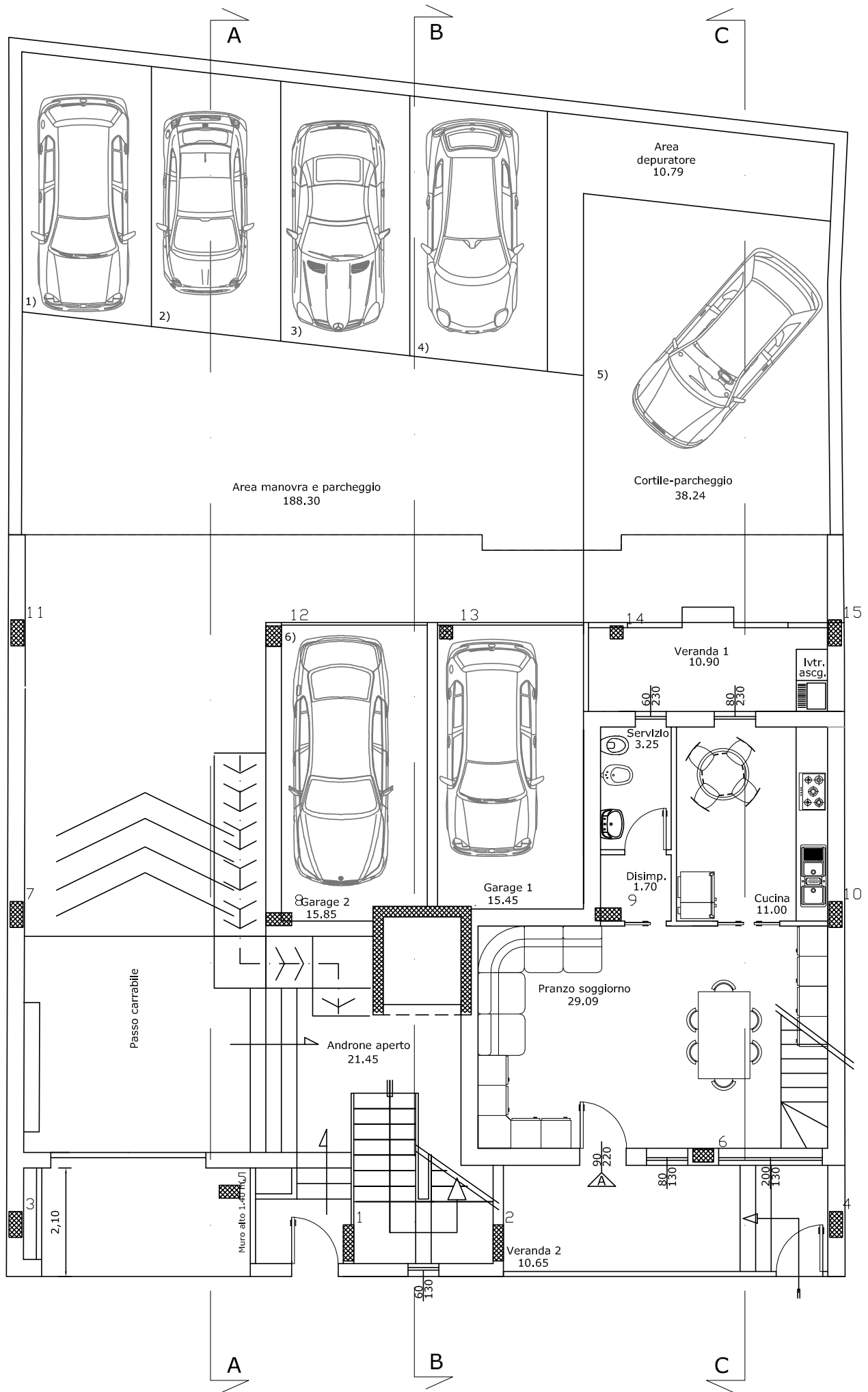
Pianta Piano terra arredata sc. 1:100
